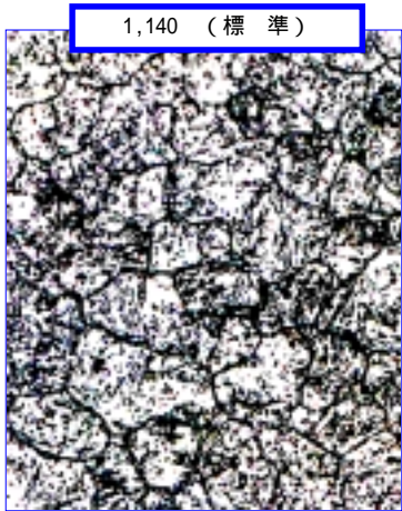
焼入れ温度と焼入れ組織 (油冷)
